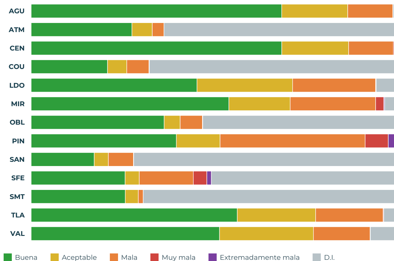
Figura 3. Horas del año según categoría de calidad del aire, por estación.
